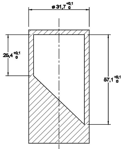
Figura 13. Cilindro para partes pequeñas
