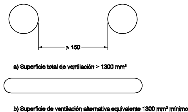
Figura 11. Ejemplo de área de ventilación alternativa
